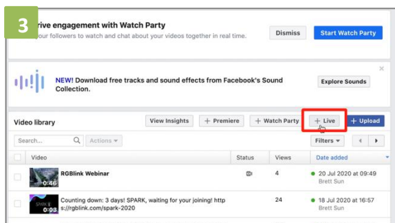
3. Click "+Live".
