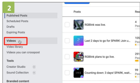
2. Click "Video".
